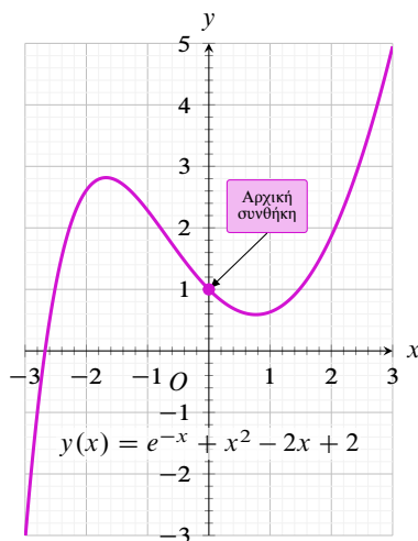
Σχήμα 2.10: Λύση του προβλήματος αρχικών τιμών.
